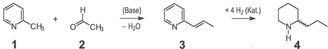
Abb. 2 Synthetische Coniin-Synthese [Breitmaier, 2008e]
