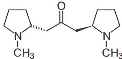
Abb. 1 Cuskygrin [Breitmaier, 2008c]
