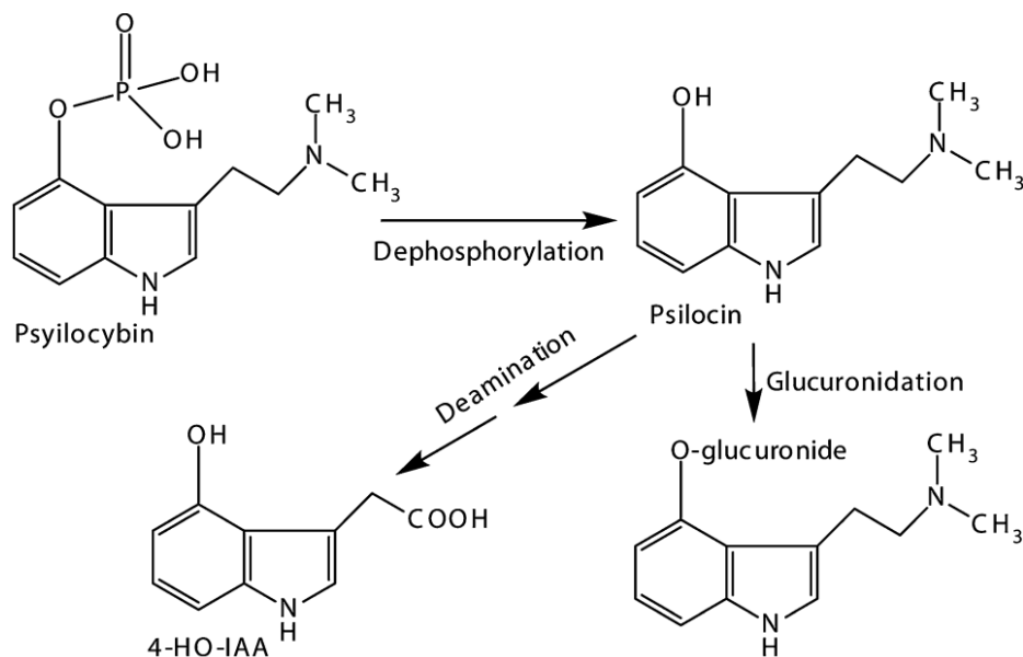
Abb. 5 Biotransformation von Psilocybin und Psilocin [Yu, 2008]
