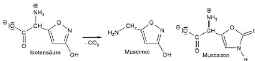
Abb. 9 Ibotensäuredecarboxylierung und Muscazonstruktur [Willmes, 2007]
