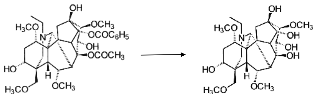
Abb. 11 Aconitin - Aconin [Breitmaier, 2008d]
