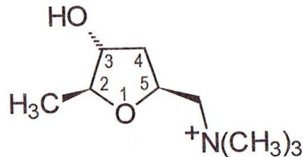
Abb. 10 (+)-Muscarin [Breitmaier, 2008d]
