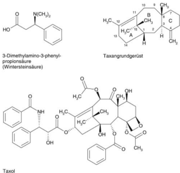
Abb. 12 Taxol [Hänsel und Sticher, 2010]
