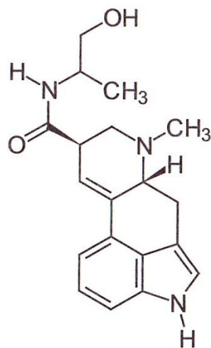
Abb. 7 (+)-Ergometrin [Breitmaier, 2008c]
