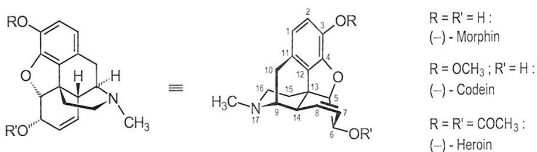
Abb. 8 Morphin, Codein, Heroin [Breitmaier, 2008c]
