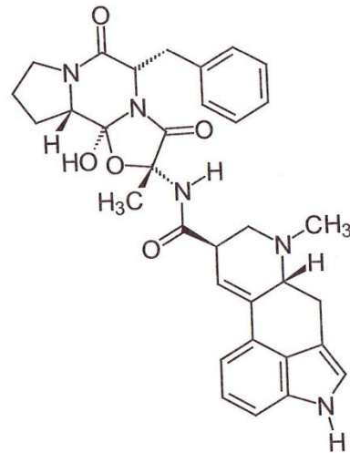
Abb. 6 (-)-Ergotamin [Breitmaier, 2008c]
