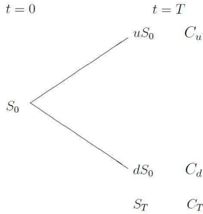
Abbildung 18: Einperiodisches Binomialmodell
