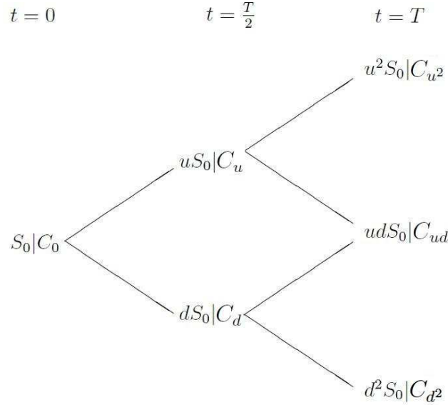
Abbildung 19: 2-Perioden-Binomialmodell
