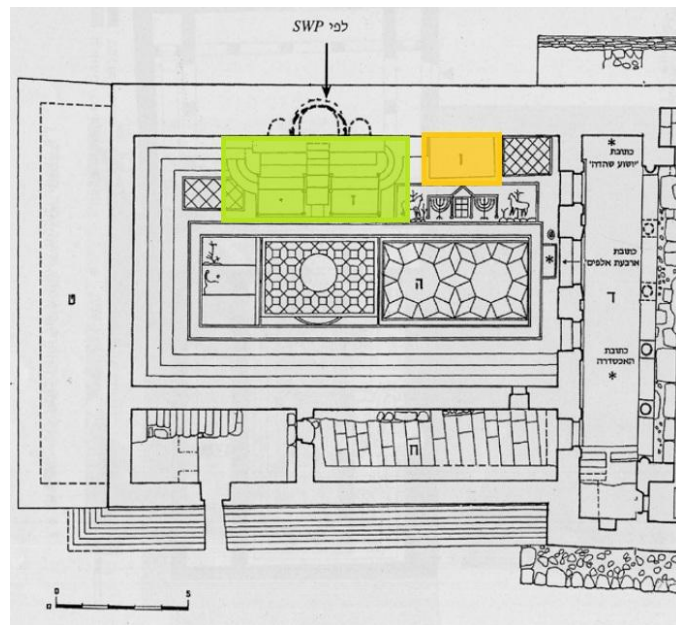
Abb. 4: Plan der Synagoge in Khirbet Susiya, genordnet (nach Z. Yeivin), der grüne Bereich stellt das zentrale bema dar und der gelbe das östliche
