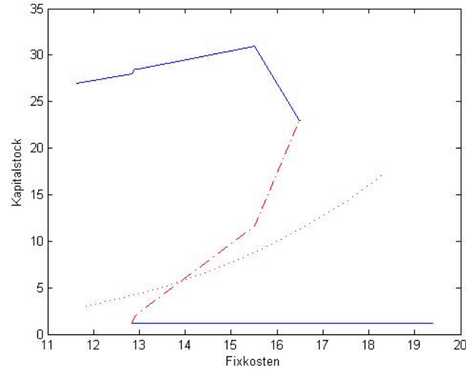
Abbildung 92: Diese Abbildung zeigt die \theta -Gleichgewichte von (48) mit den Parametern \gamma = 0.25 , A = 1 , B = 10 , \rho = 0 , \alpha = 1 und p = \sqrt[3]{\frac{85}{100}} .
