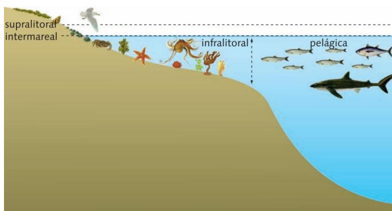
Ilustración 14. la zonación del mar en profundidad
