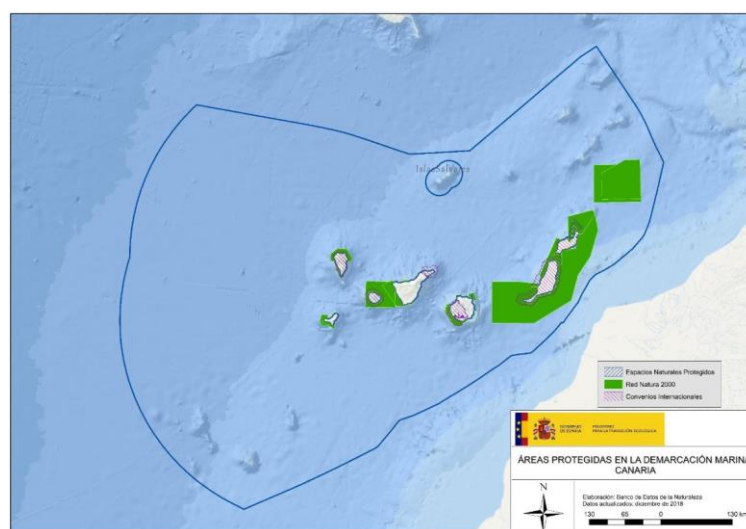
Ilustración 3. demarcación marina de Canarias
