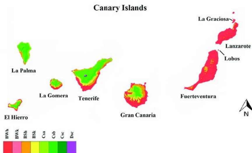
Ilustración 6. clasificación climática de Köppen-Geiger de las islas Canarias
