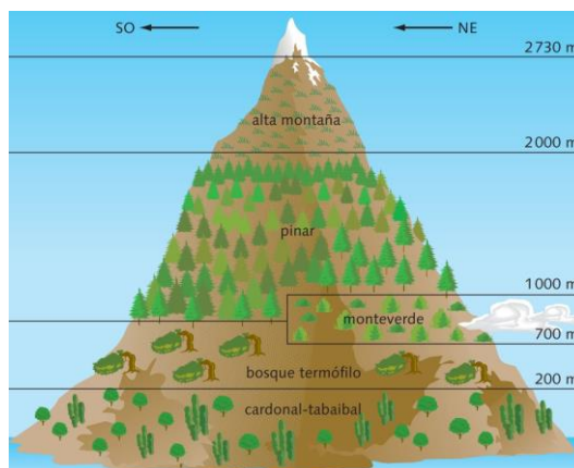
Ilustración 13. pisos de vegetación
