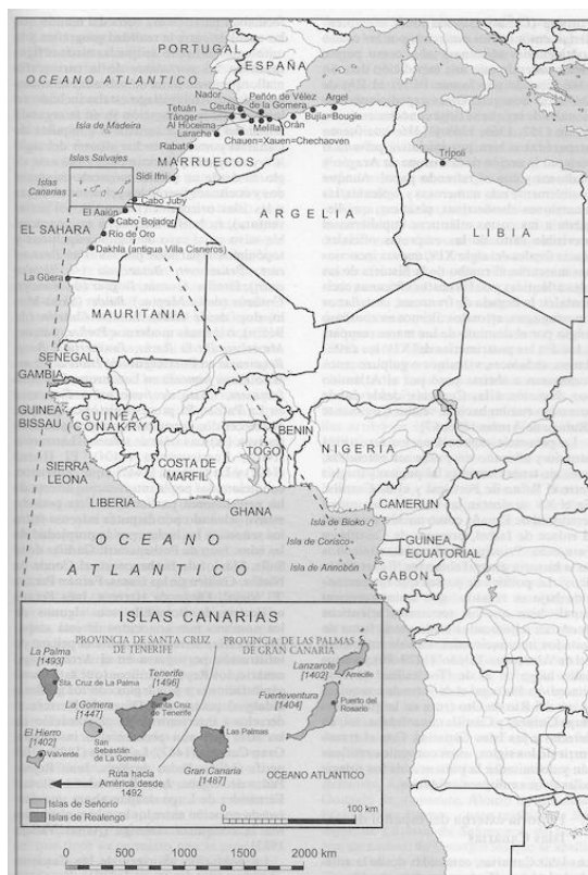
Ilustración 1. localización de las islas Canarias
