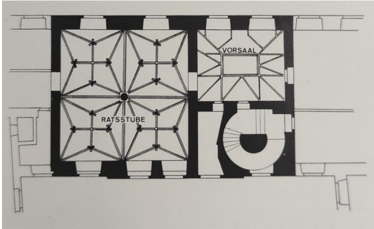
Abb. 13: Altes Rathaus, Grundriss der Ratsstube mit Vorsaal im 1. Obergeschoß des Nordtraktes gegen die Salvatorgasse.
