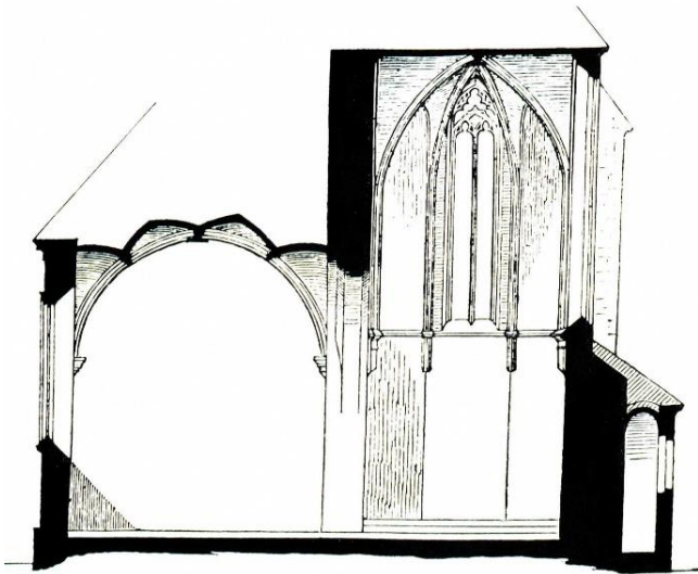
Abb. 10: Wien, St. Salvator, Querschnitt durch beide Kapellen, nach Karl Lind.
