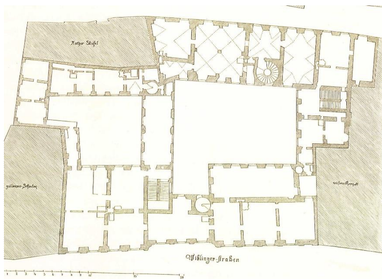
Abb. 22: Altes Rathaus, Grundriss aus dem Jahr 1751, der Arkadengang im Hof wurde zu einem Quertrakt ausgebaut.
