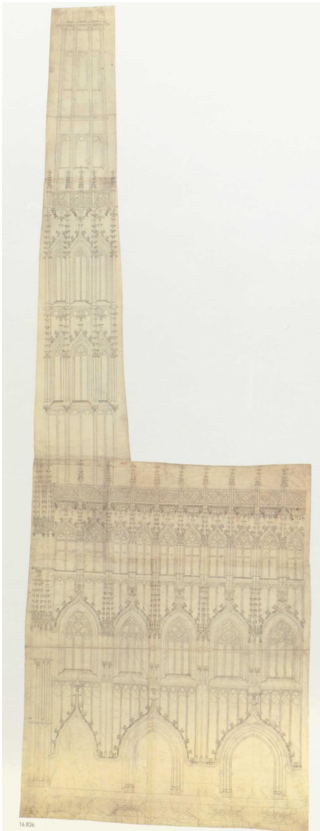
Abb. 54: Laurenz Spenning zugeschrieben, Riss 16.836r, Fassadenaufriss eines Sakralbaus (Marien- bzw. Salvatorkapelle), Reißfeder auf Pergament, 2. H. 15. Jh., Aufbewahrungsort
