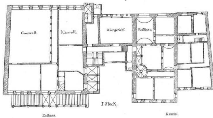
Abb. 72: Rathaus, Bern, Grundriss des 1. Obergeschoßes.
