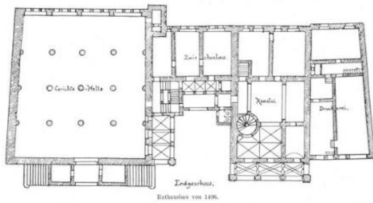
Abb. 71: Rathaus, Bern, Grundriss des Erdgeschoßes.
