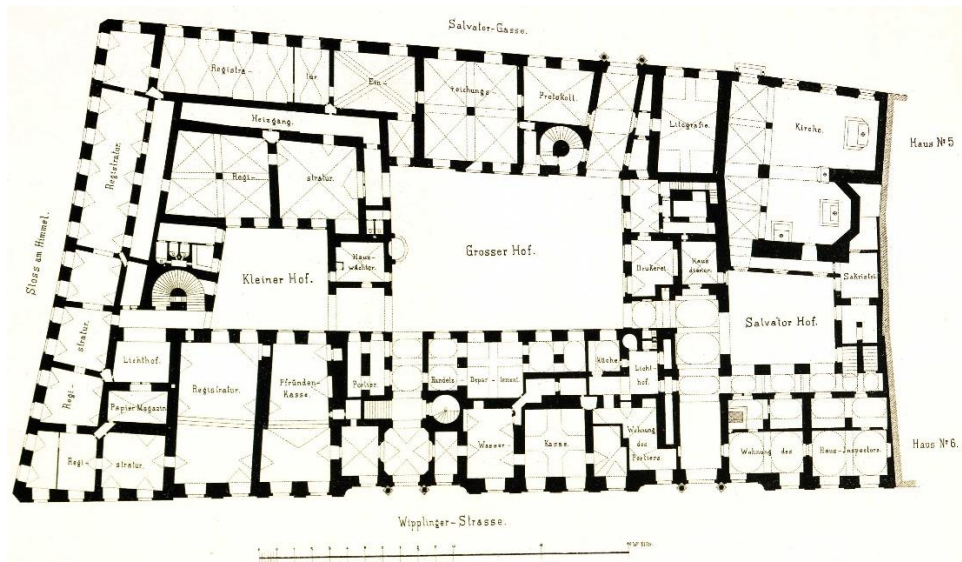
Abb. 66: Altes Rathaus, Grundriss des alten Rathauses im Erdgeschoß, 1883.
