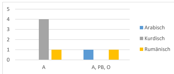
Abb. 22 – Abweichungen bei Testelement /j/ vs. /ç/ nach L1 und Testebene
