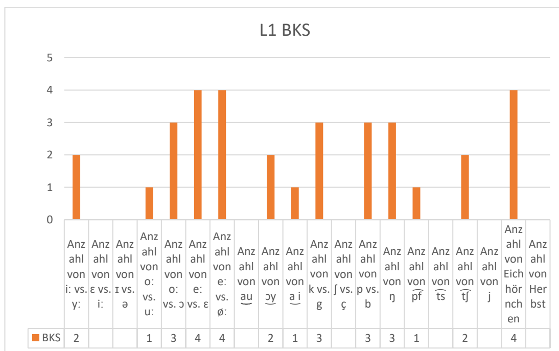
Abb. 30 – Abweichungen bei L1 BKS
