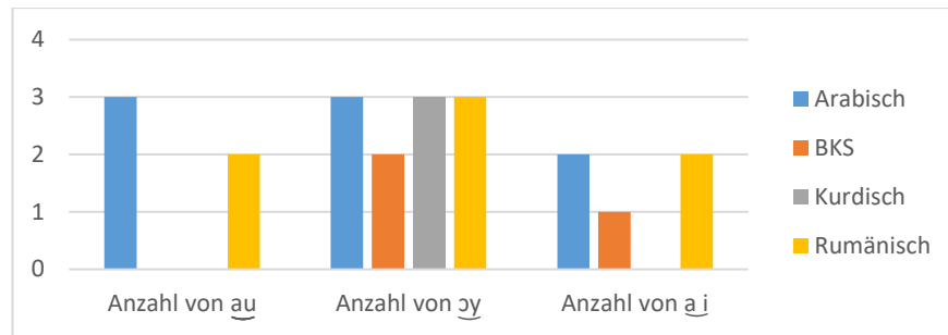
Abb. 16 – Abweichungen bei den Testelementen au , ɔy und a i nach L1
