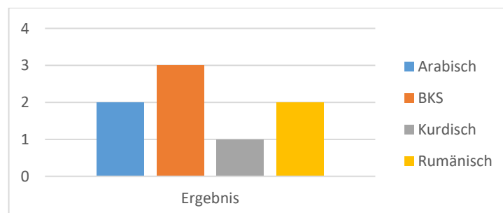
Abb. 25 – Abweichungen bei Testelement /\eta/ nach L1
