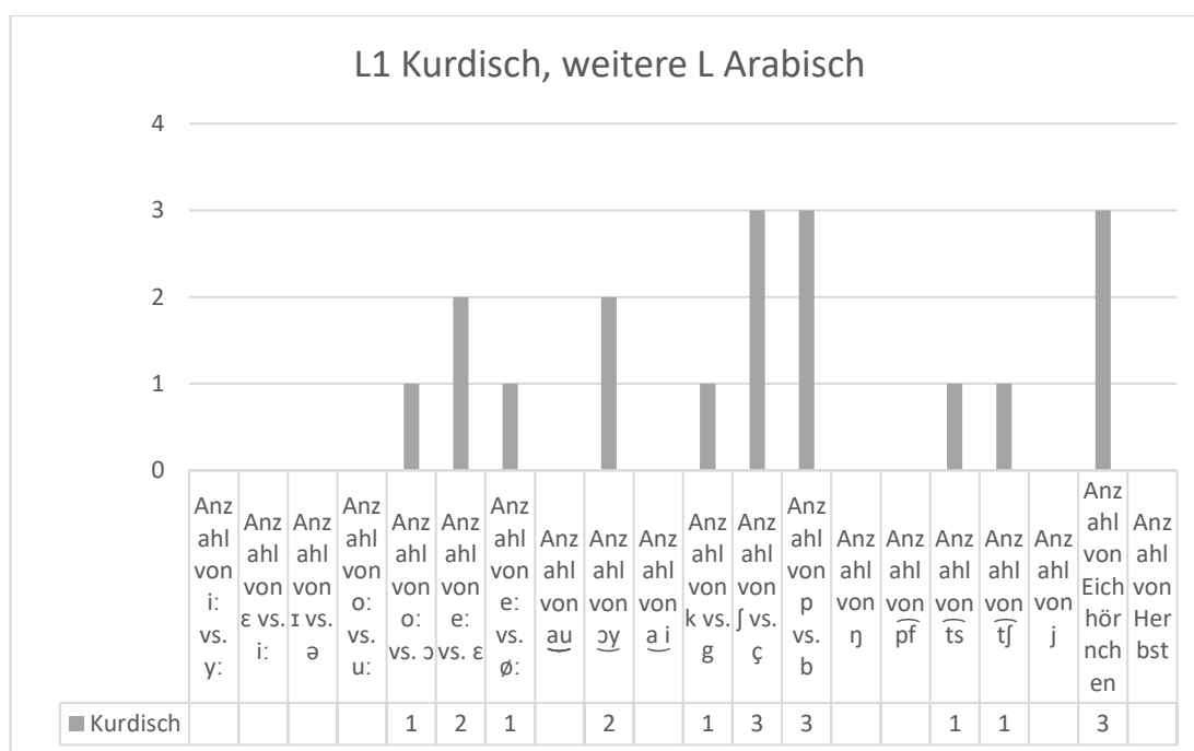
Abb. 32 – Abweichungen bei L1 Kurdisch und Arabisch als weitere L
