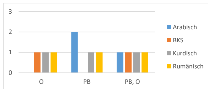
Abb. 17 – Abweichungen bei Testelement ɔy nach L1 und Testebene
