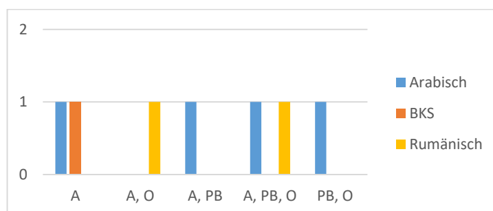
Abb. 23 – Abweichungen bei Testelement /pf/ nach L1 und Testebene
