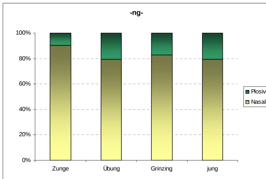
Abbildung 26: Häufigkeitsverteilung -ng-
