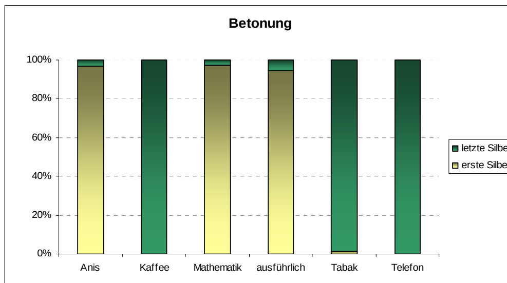
Abbildung 33: Häufigkeitsverteilung Betonung
