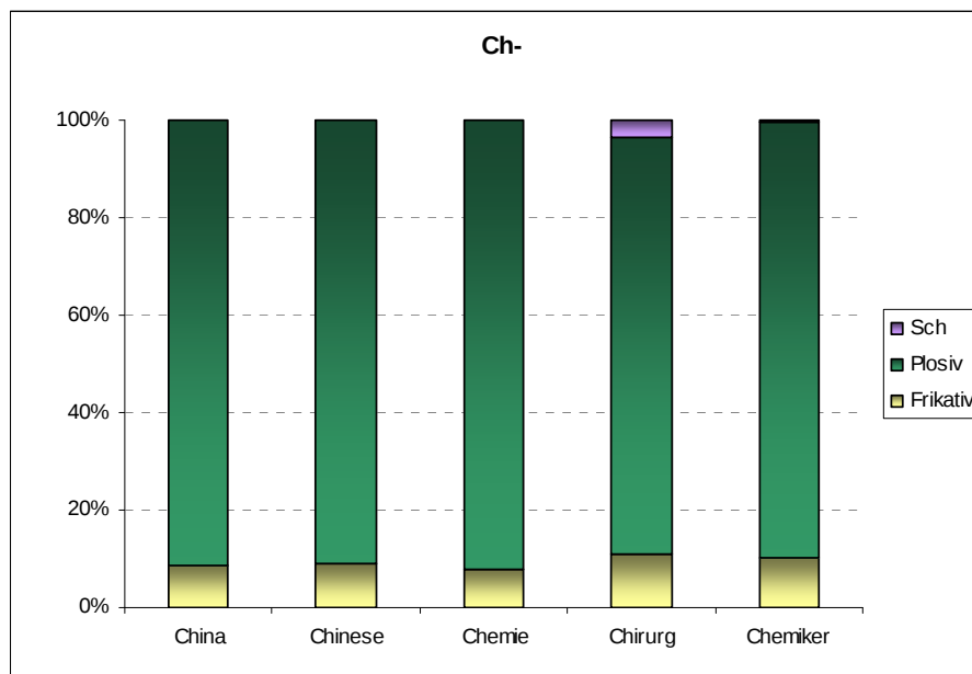
Abbildung 24: Häufigkeitsverteilung ch-
