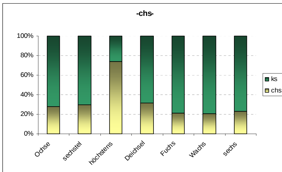
Abbildung 28: Häufigkeitsverteilung -chs-
