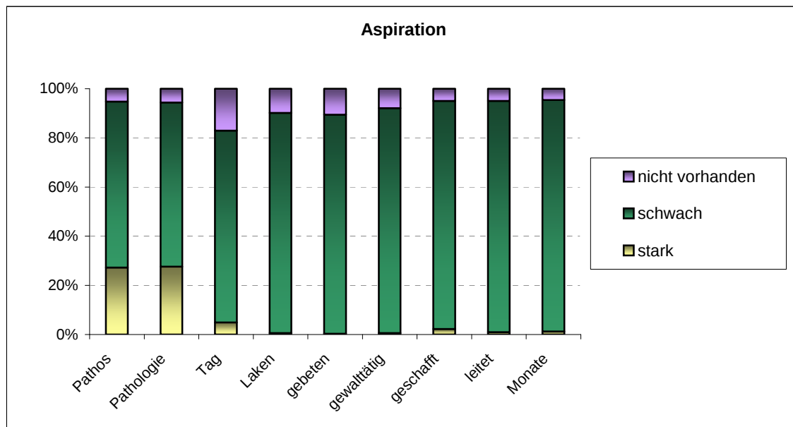
Abbildung 20: Häufigkeitsverteilung Aspiration
