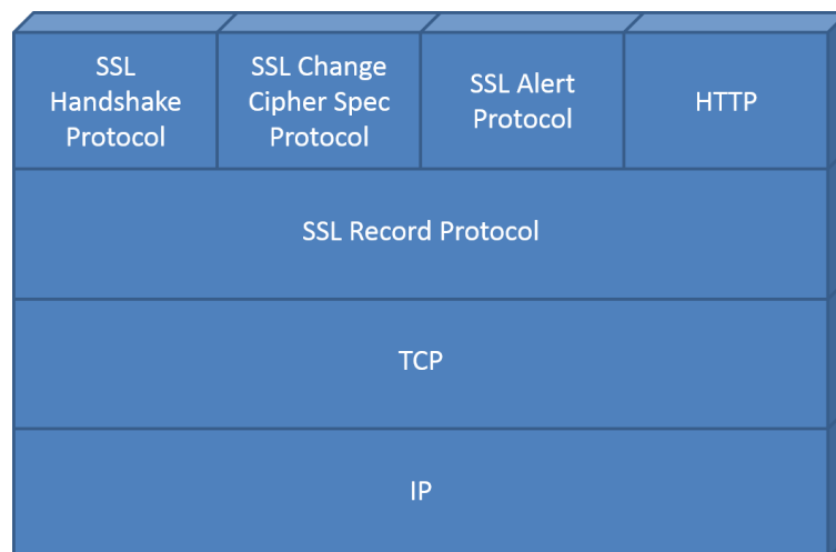
Abbildung 28: SSL-Protocol-Stack
