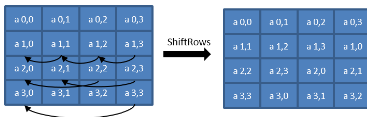
Abbildung 20: ShiftRows
