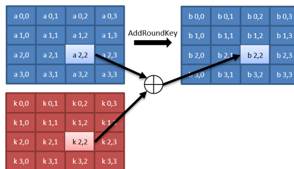
Abbildung 18: AddRoundKey
