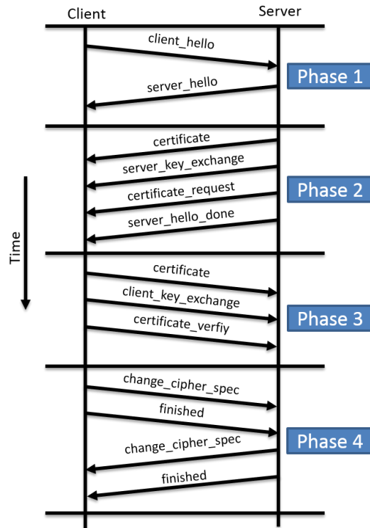
Abbildung 30: Handshake-Protocol-Action
