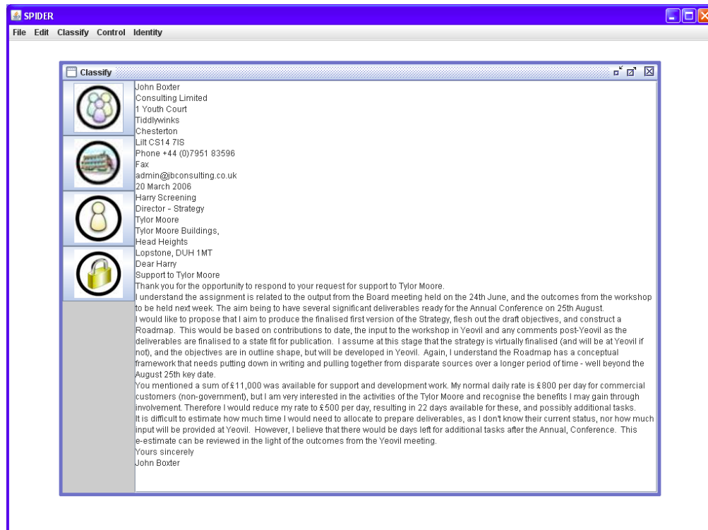
Abbildung 78: SPIDER-Projekt – Konzept
