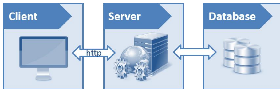
Abbildung 14: eSprint-3-Tier-Architektur (Überblick)
