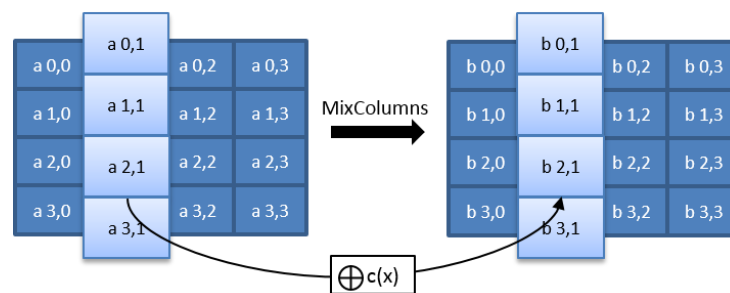
Abbildung 21: MixColumns
