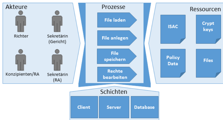
Abbildung 47: Übersicht – Prozesslandschaft
