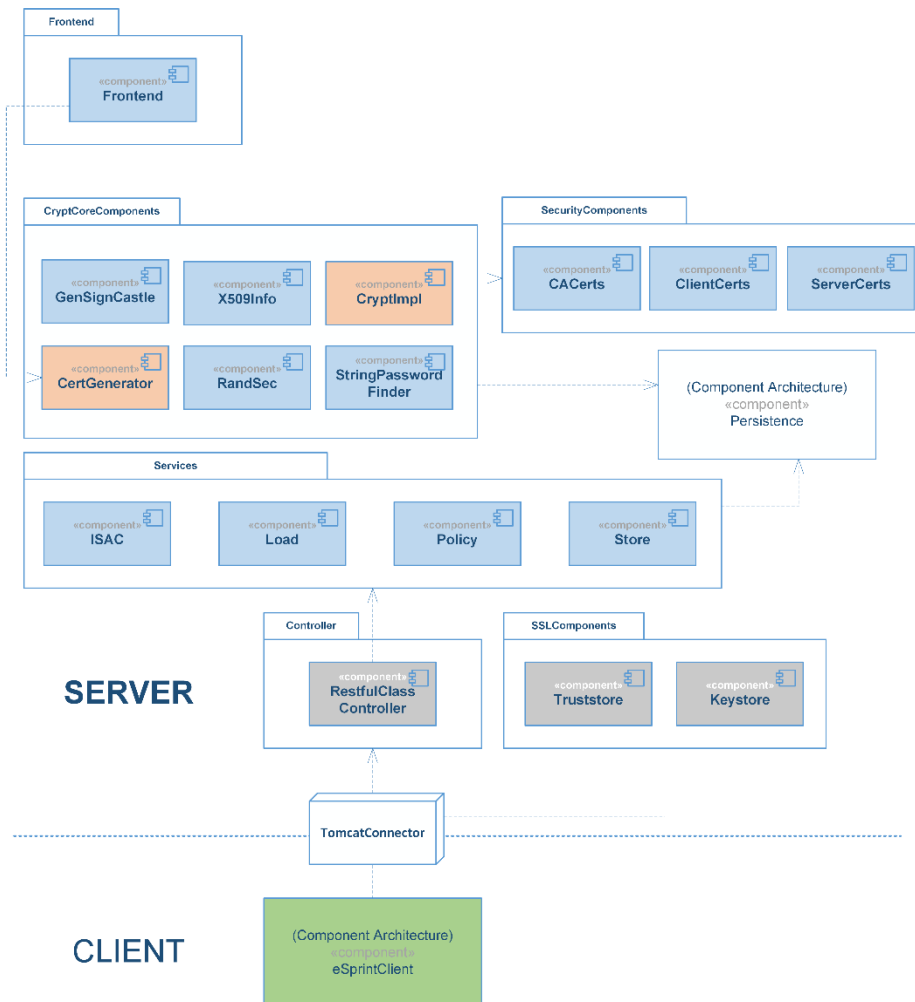
Abbildung 45: Komponentendiagramm – Server
