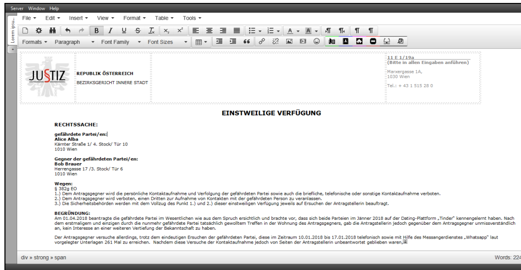
Abbildung 70: Überblick – eSprint-Client
