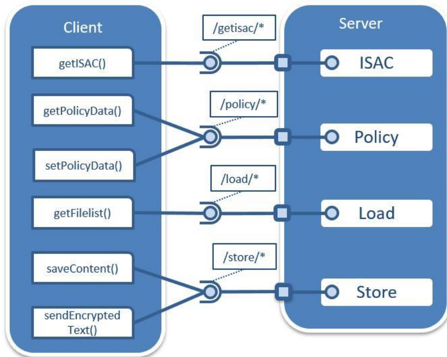
Abbildung 57: Schnittstellendefinition
