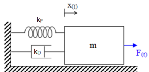
Abb.56: Feder-Dämpfung Kombination
