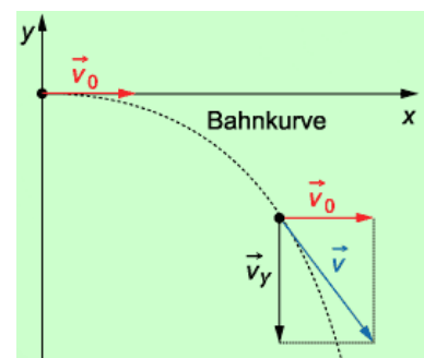
Abb.49: Waagrechter Wurf
