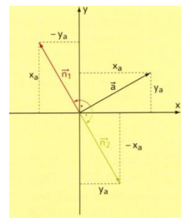
Abb.40: Normalvektoren
