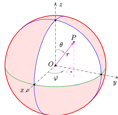
Abb.35:Kugelkoordinatensystem
