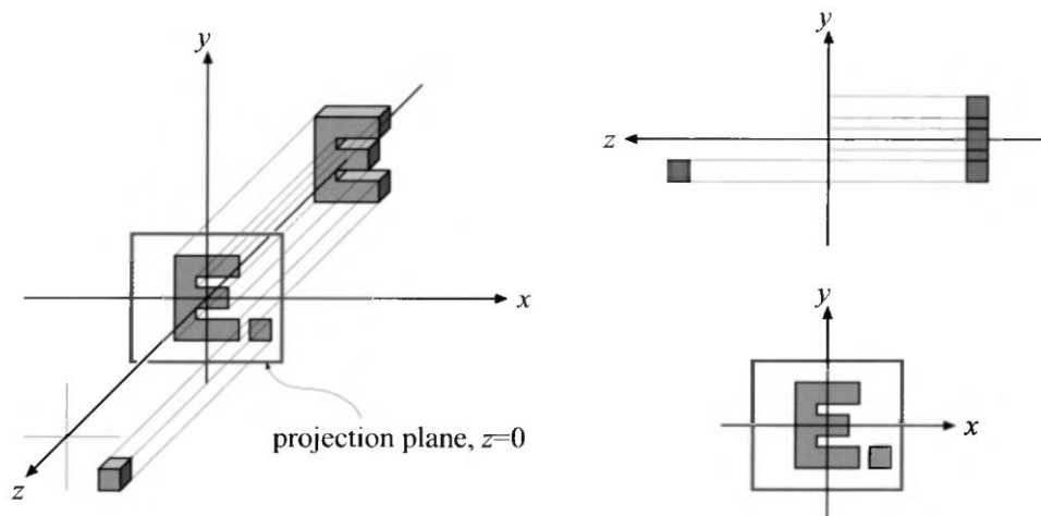
Abb.79: Orthogonale Projektion
