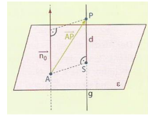
Abb.46: Abstand Punkt-Ebene
