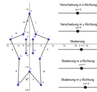
Abb.115: Skalierungsfaktor s_y = 2
