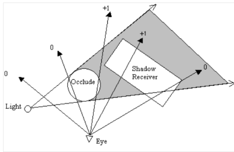
Abb.93: Tiefenpass-Test
