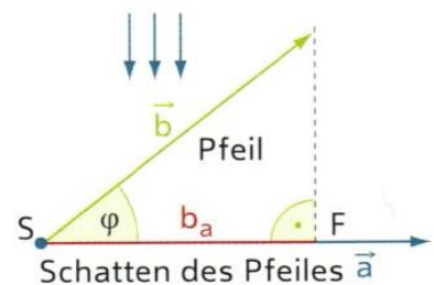
Abb.39: Normalprojektion
