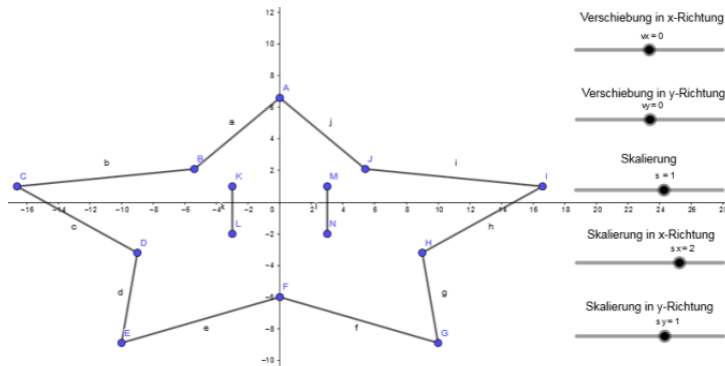
Abb.114: Skalierungsfaktor s_x = 2
