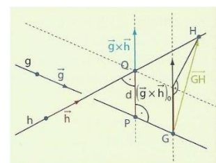
Abb.45: Abstand Gerade-Gerade
