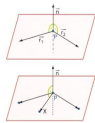
Abb.43: Normalvektorform
