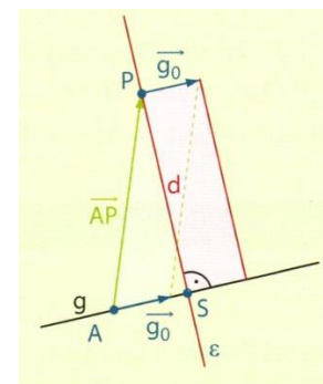
Abb.44: Abstand Punkt-Gerade
