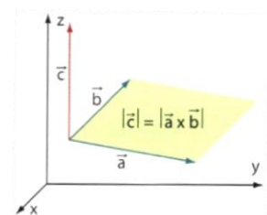
Abb.41: Kreuzprodukt
