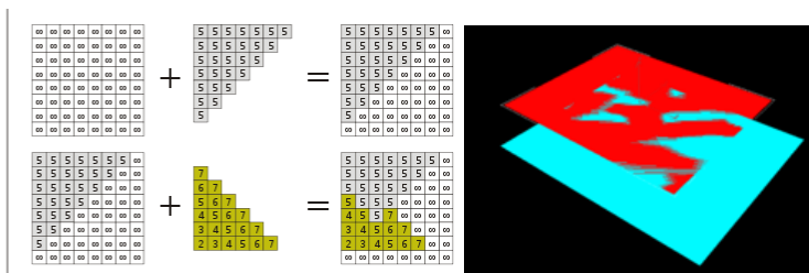
Abb.81: Prinzip des z-Buffers
