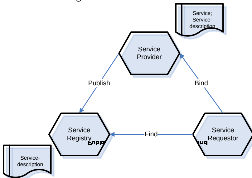
Abbildung 2: Operationen und Rollen in SOA 12
