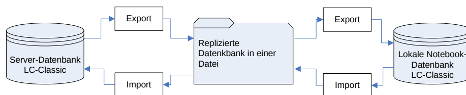
Abbildung 13: mobile Auftragserfassung "offline"
