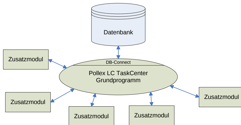
Abbildung 8: Struktur TaskCenter
