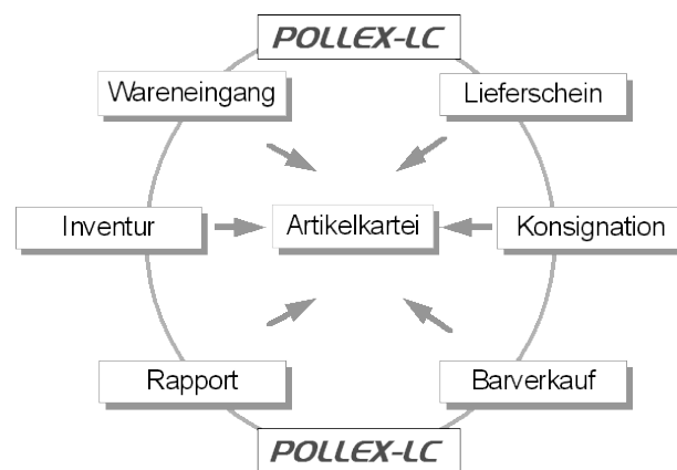
Abbildung 10: Einflussfaktoren Artikelkartei 59
