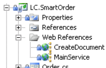
Abbildung 28: Webservicereferenzierung
