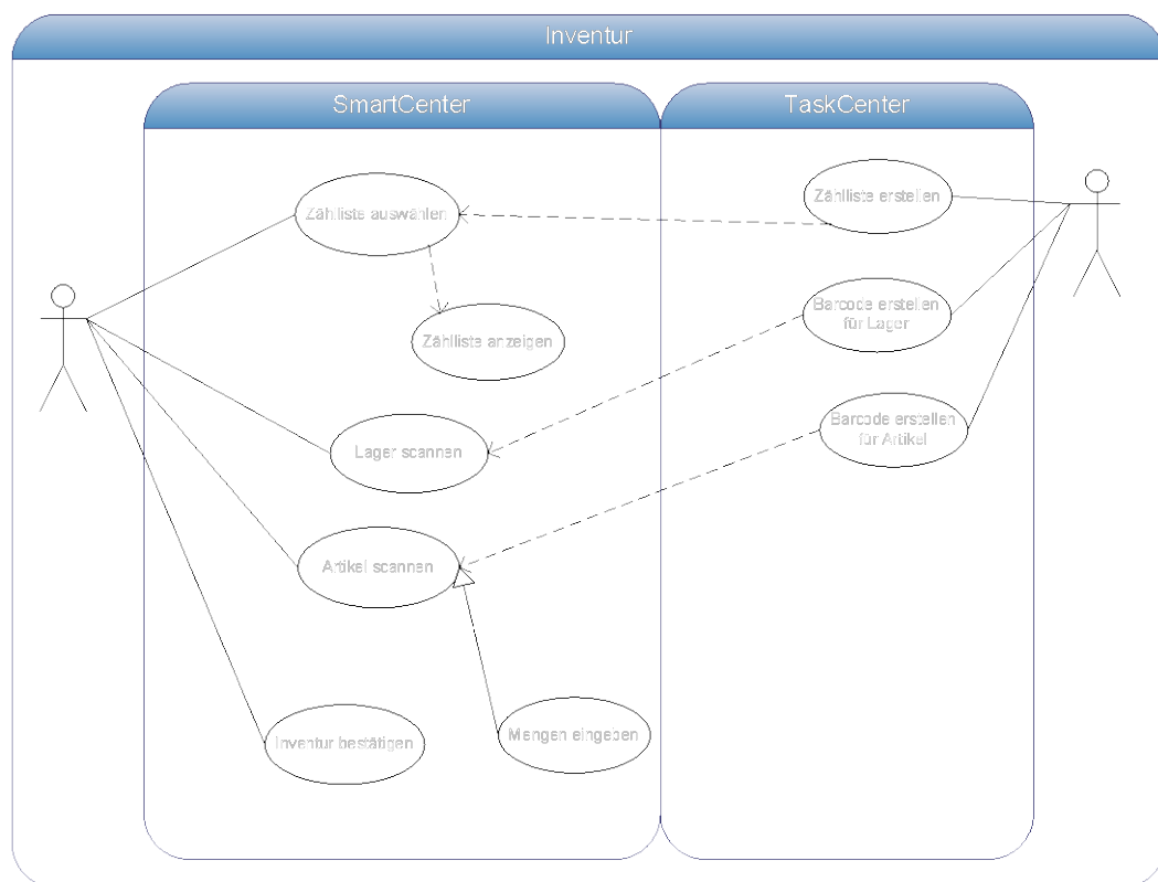
Abbildung 22: Anwendungsfalldiagramm Inventur
