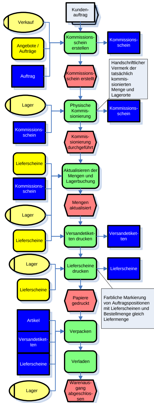
Abbildung 17: Prozess Warenausgang
