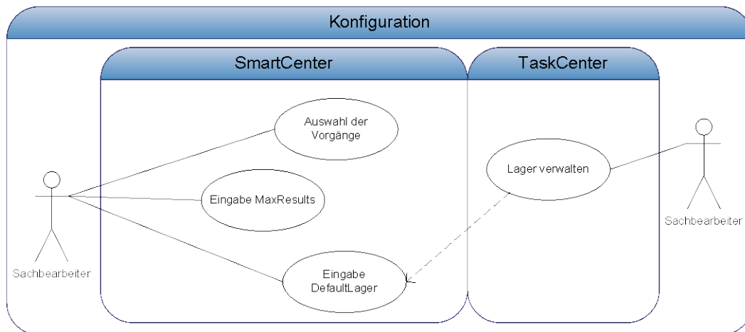
Abbildung 21: Anwendungsfalldiagramm Konfiguration
