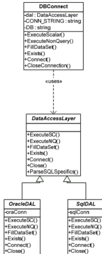
Abbildung 27: Datenbankzugriff vereinfacht 84
