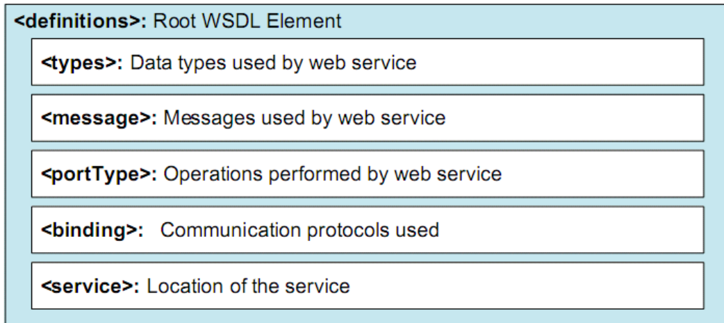
Abbildung 3: Aufbau eines WSDL Dokuments 15
