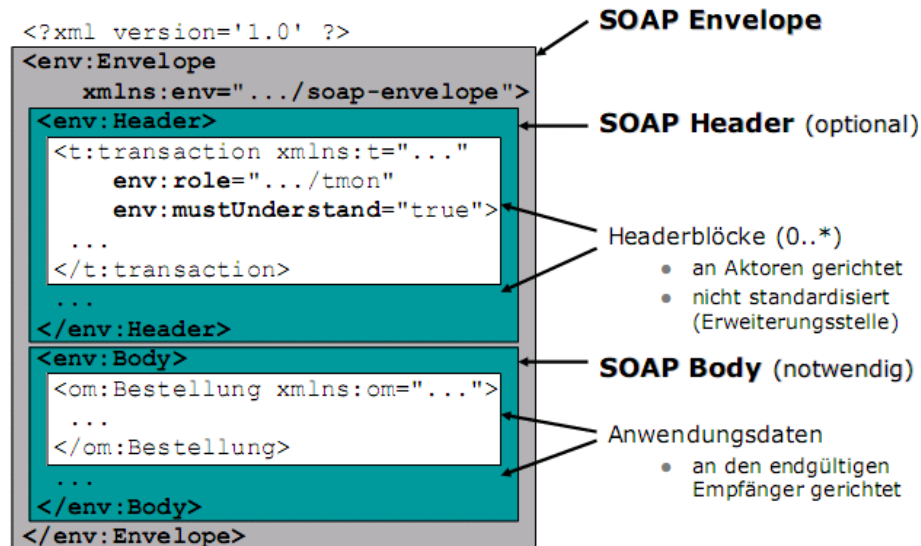
Abbildung 4: Bestandteile von SOAP 27
