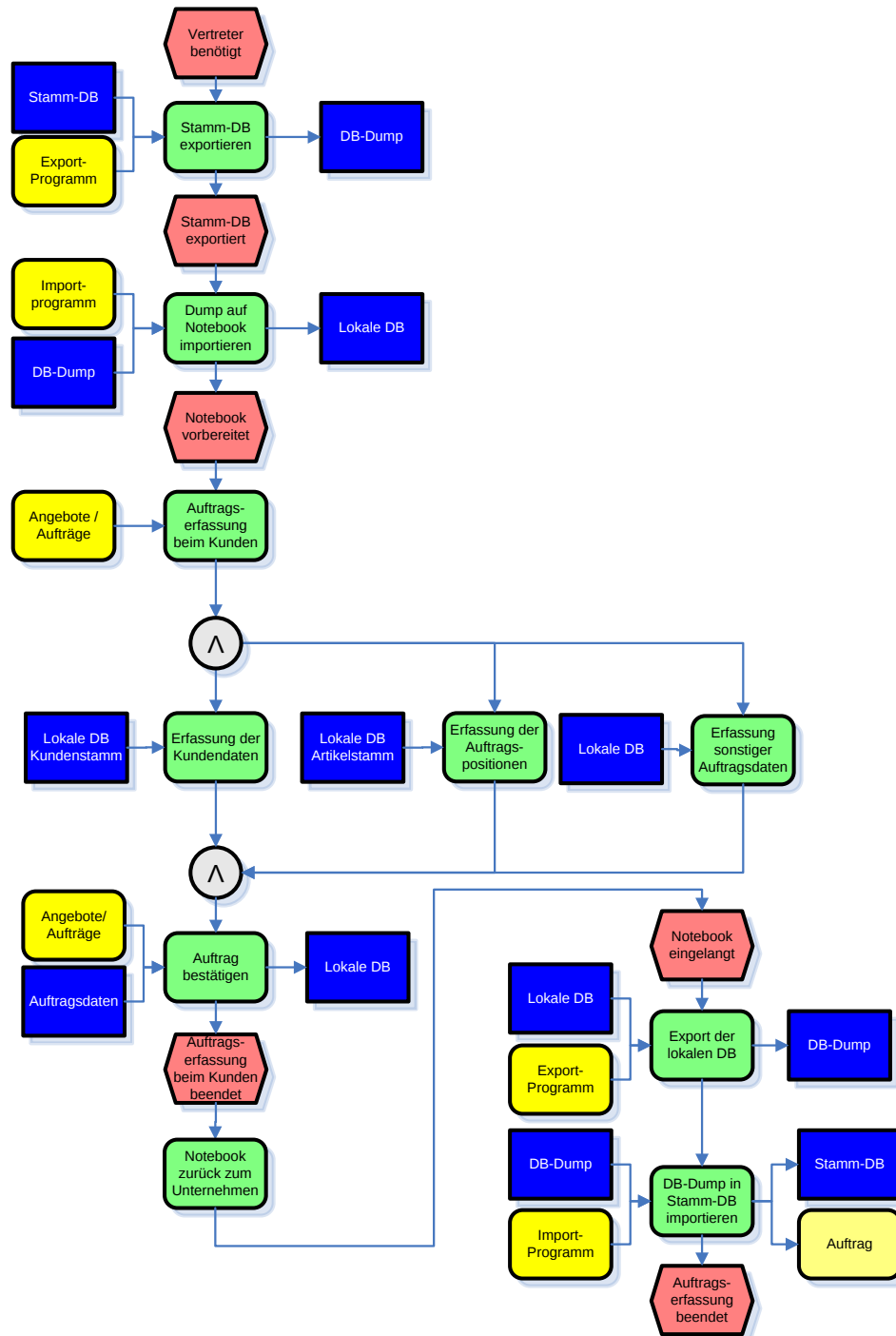
Abbildung 14: Prozessablauf der mobilen Auftragserfassung
