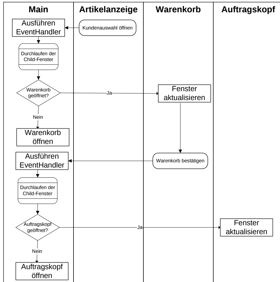
Abbildung 30: Beispiel für Eventhandling 89
