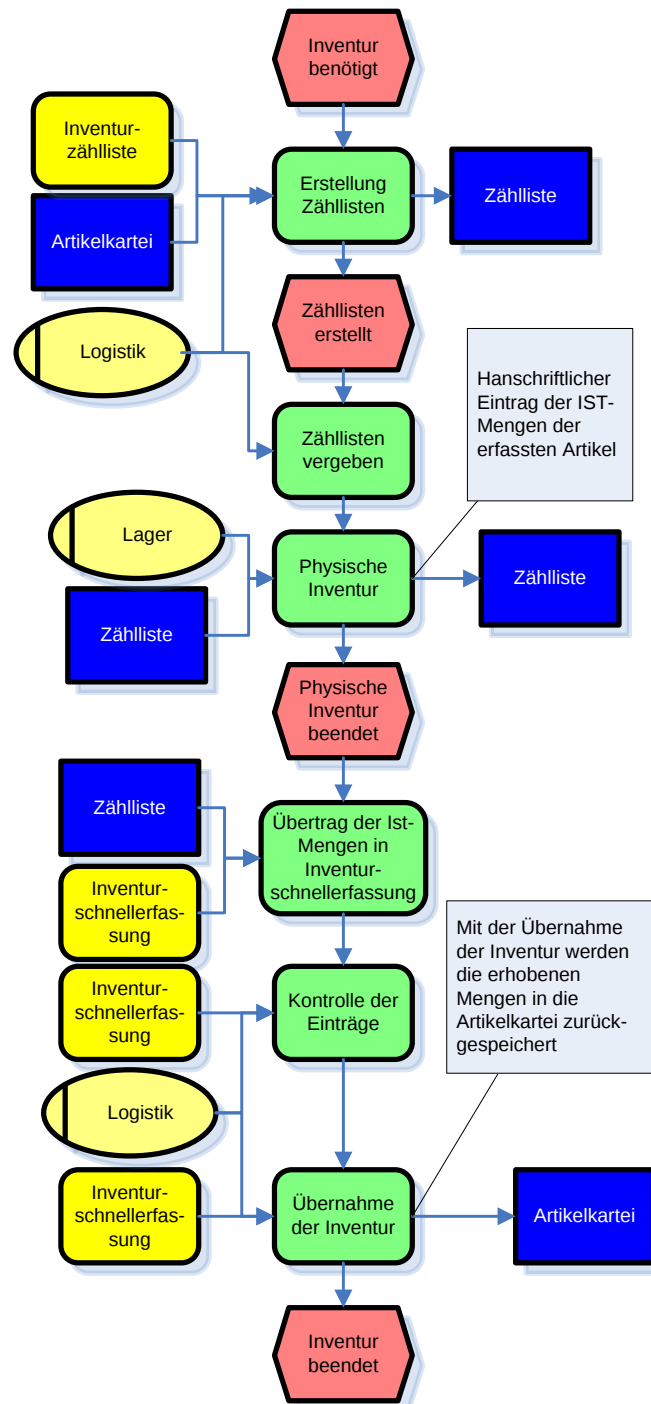
Abbildung 15: Prozessablauf Inventur
