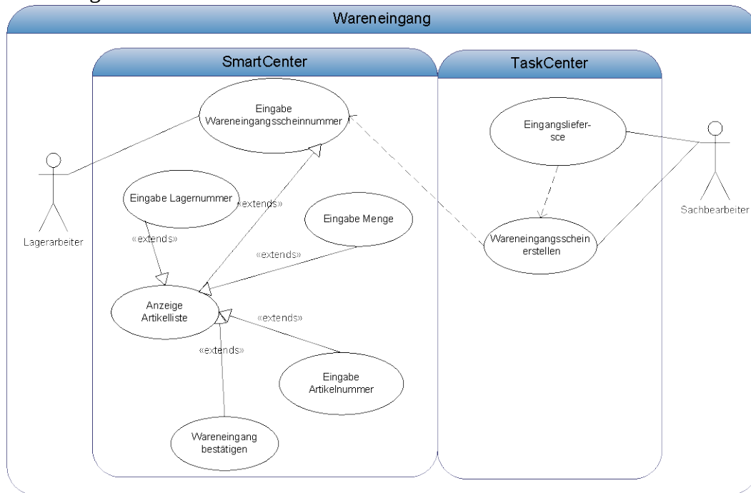
Abbildung 23: Anwendungsfalldiagramm Wareneingang
