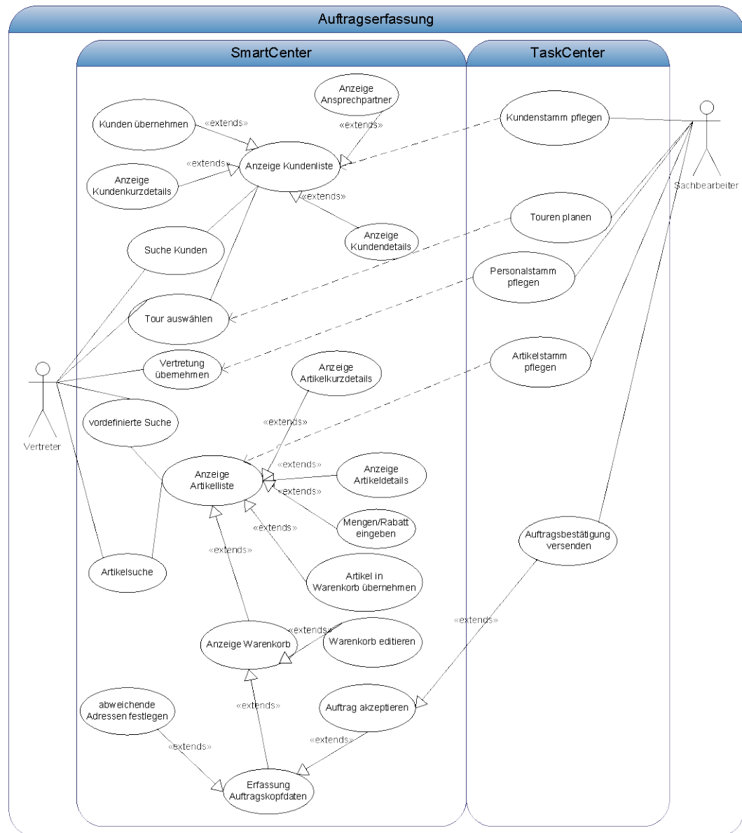
Abbildung 25: Anwendungsfalldiagramm Auftragserfassung
