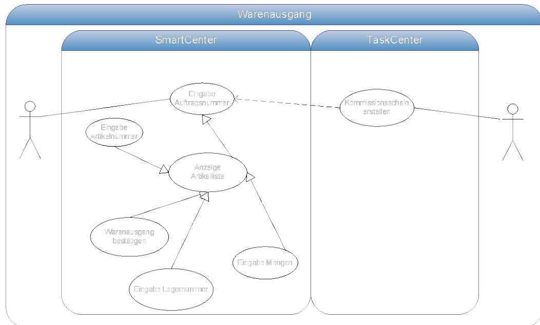
Abbildung 24: Anwendungsfalldiagramm Warenausgang
