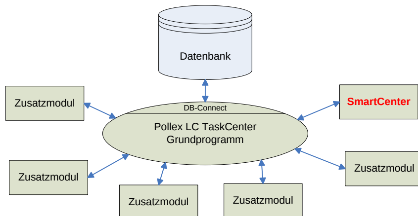
Abbildung 19: Modul SmartCenter
