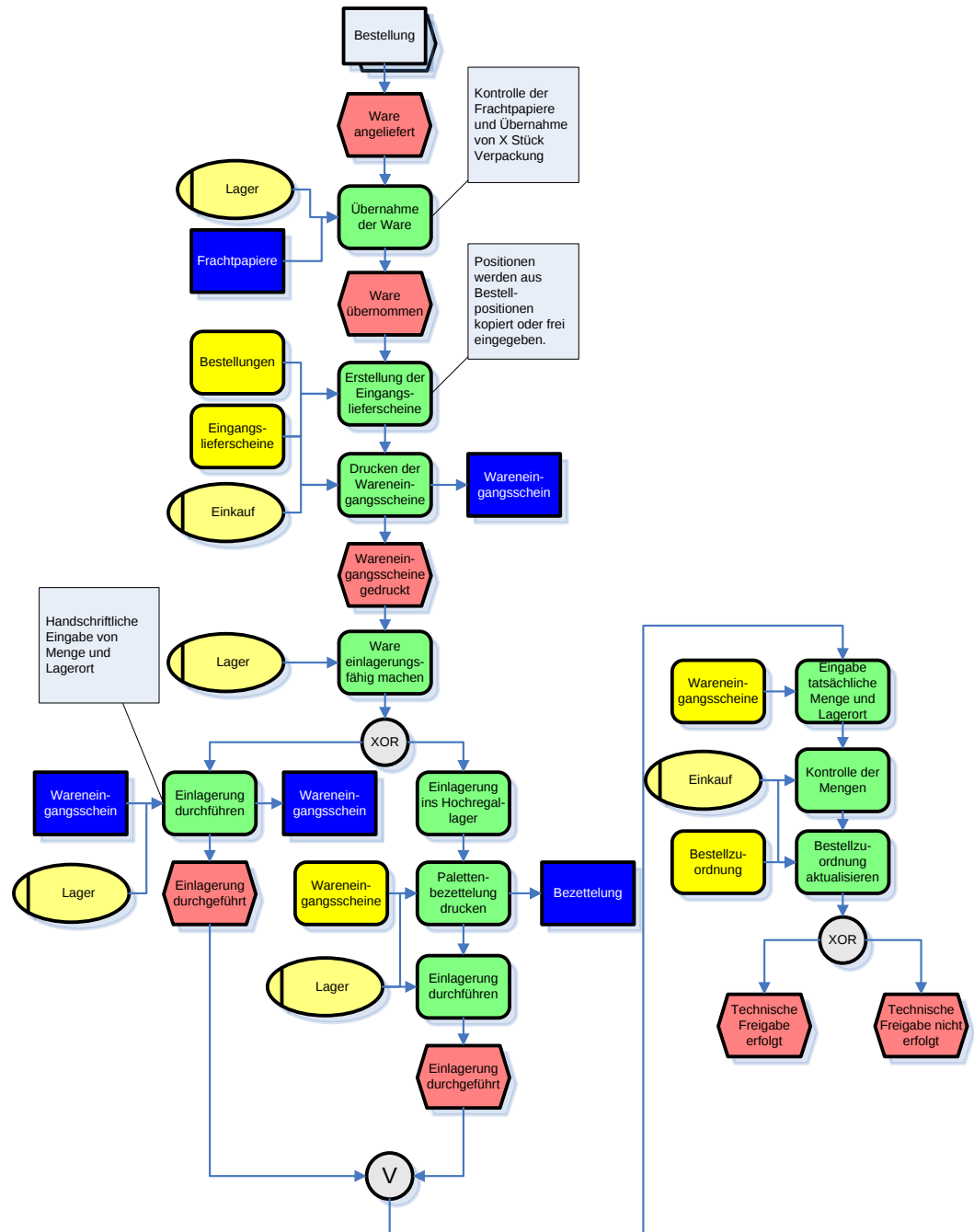
Abbildung 16: Prozess Wareneingang
