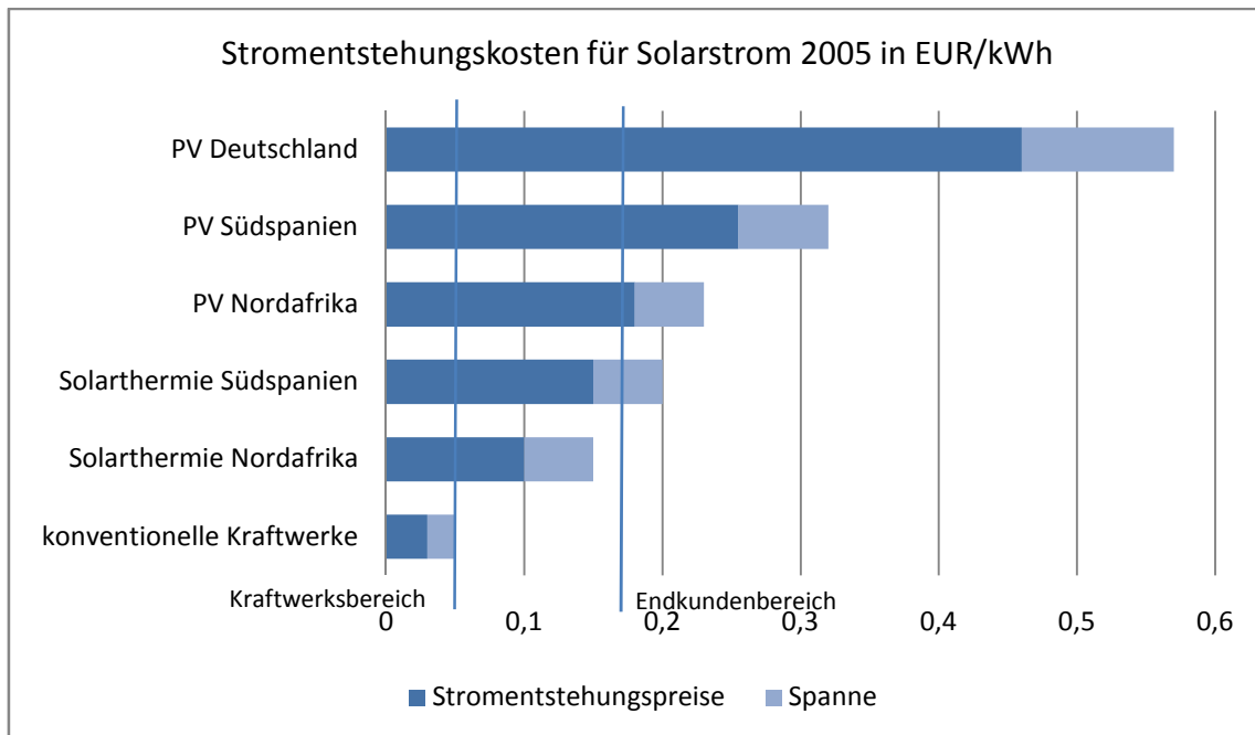
Abbildung 18 Stromentstehungskosten aus Solarstrom, (Quaschnig, 2005)
