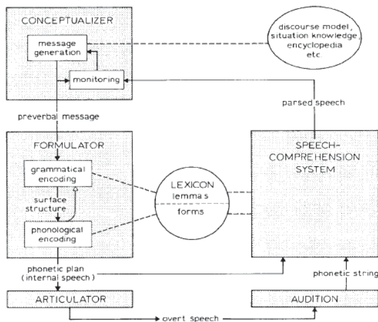
Abb. 2: Der Sprachproduktionsprozess nach Levelt (1989:9)
