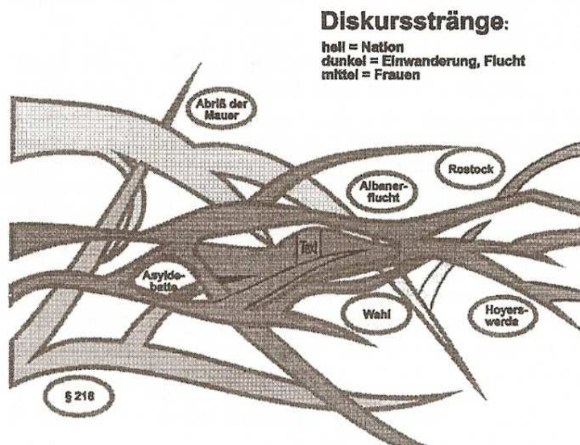
Ilustración 2 Modelo de fases del discurso
