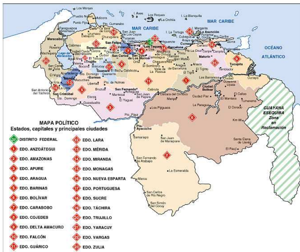
Ilustración 4 Mapa político de Venezuela
