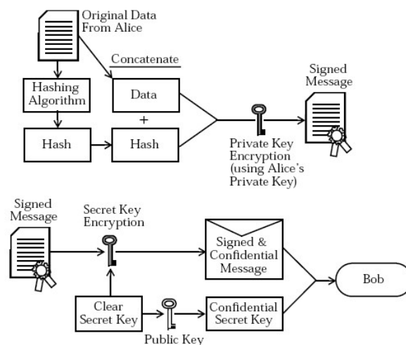
Abbildung 4.4: Alices Schritte zum Verschlüsseln und Hashen der Nachricht
