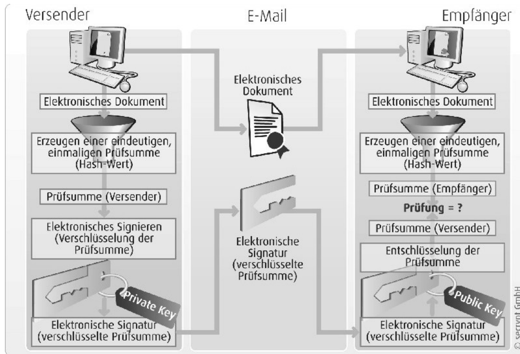
Abbildung 3.1: Datenfluss beim Erzeugen digitaler Signaturen
