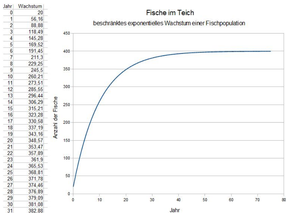
Abbildung 2.3.2: „Fische im Teich“ bei beschränktem exponentiellen Wachstum
