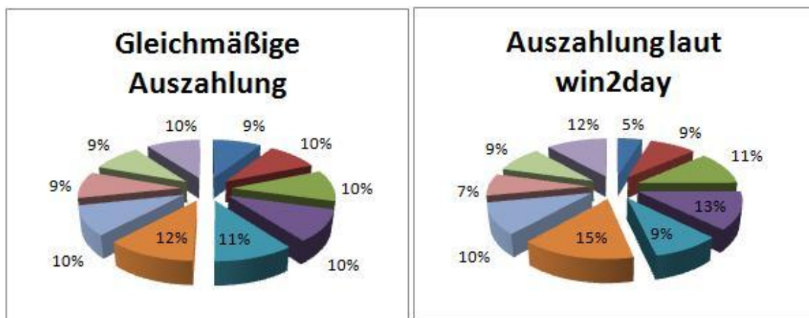
Abbildung 39: Auszahlungsvergleich ZufallsKI
